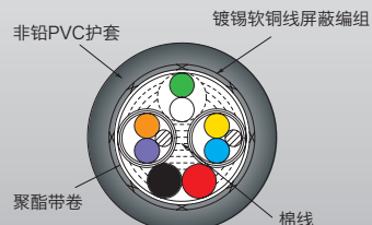
电缆规格构造图 (标准品)
